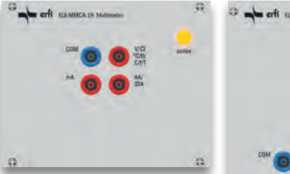
Zusatzsteckschub mit Alufont für Digitalmultimeter und Leistungsmesser 28 TE / 113 mm Zur Aufnahme von 1 Digitalmultimeter EL6.D oder 1 Leistungsmesser inkl. Digitalmultimeter EL6.P. Ansteuerung durch Steuerzentrum über rückseitigen e-Bus. Eingänge: 4 SLB 1 für alle Messgrößen Anzeige: RGB-LED für Gerät active
