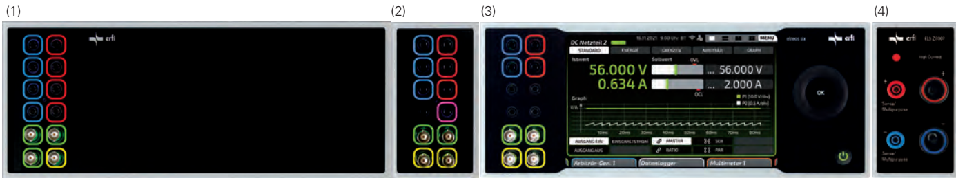
Gerätekombination mit verschiedenen Zusatzeinschüben (1) Zusatzeinschub mit weiterem Digitalmultimeter, Funktionsgenerator und Doppelnetzteil 2 x 0-32 V / 2 A und (2) Zusatzeinschub mit Digitalmultimeter und Leistungsmesser. (3) Steuerzentrum mit 1 Powernetzteil 0-32 V / 50 A und (4) Zusatzeinschub Hochstromoutlet.
