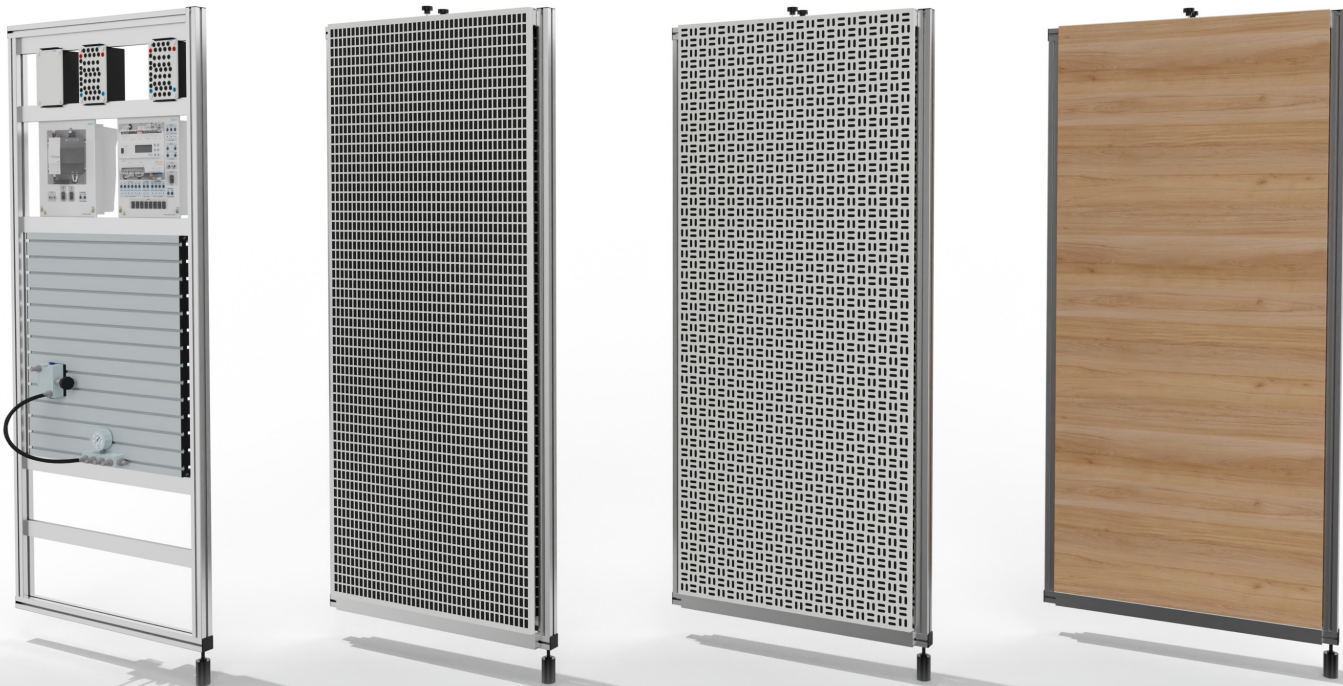
Außentür mit 5 H-Schienen zur Aufnahme von z. B. Festo Didactic SE ER-Komponenten, DIN A4-Lehrmitteln und einer Aluminium-Profilplatte für Festo Pneumatik-Komponenten Außentür mit Lochblech, Rechtecklochung Außentür mit Lochblech, Ovallochung Außentür mit Tischlerplatte
